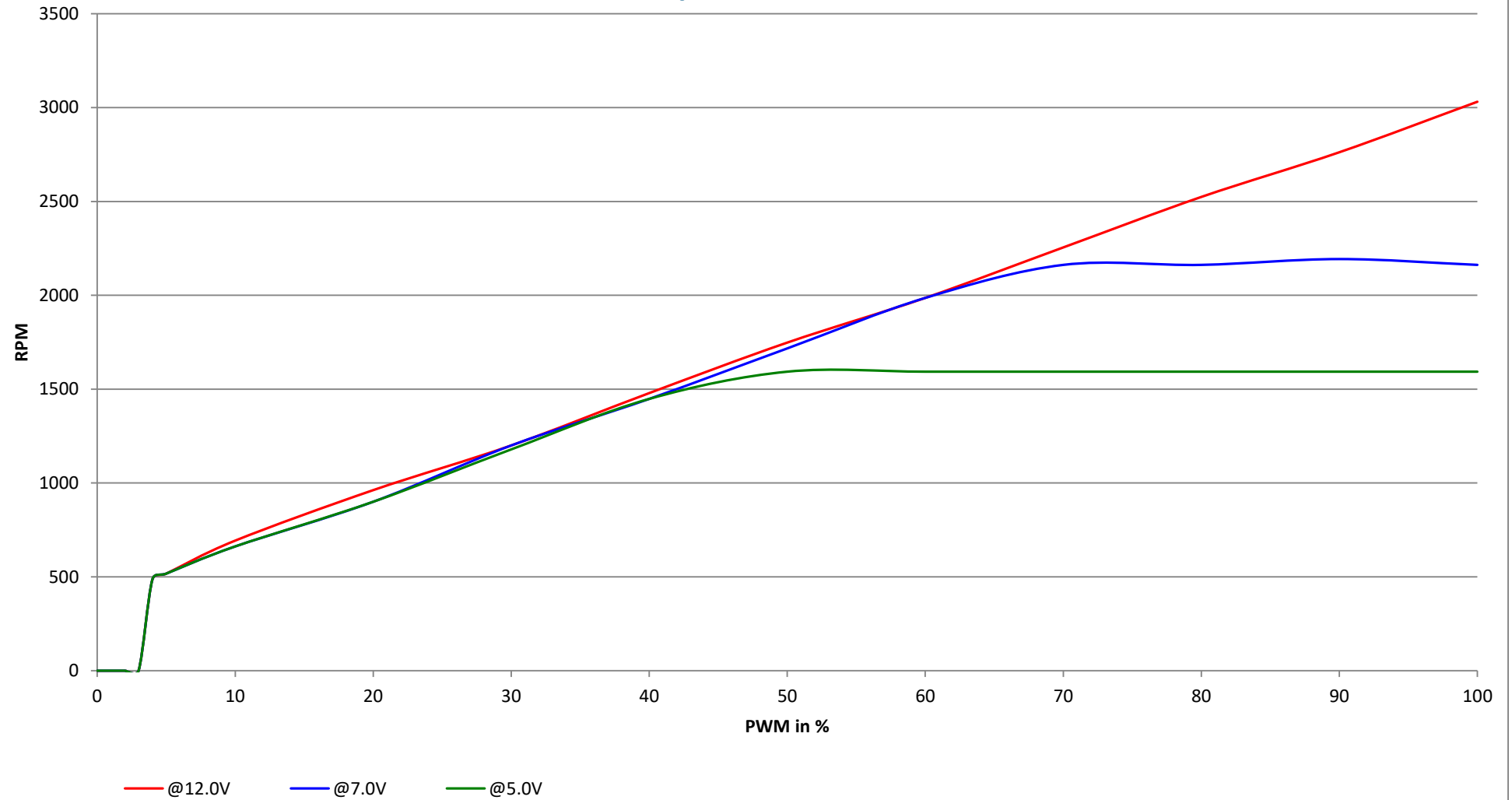
Fan Speed Vs. PWM
